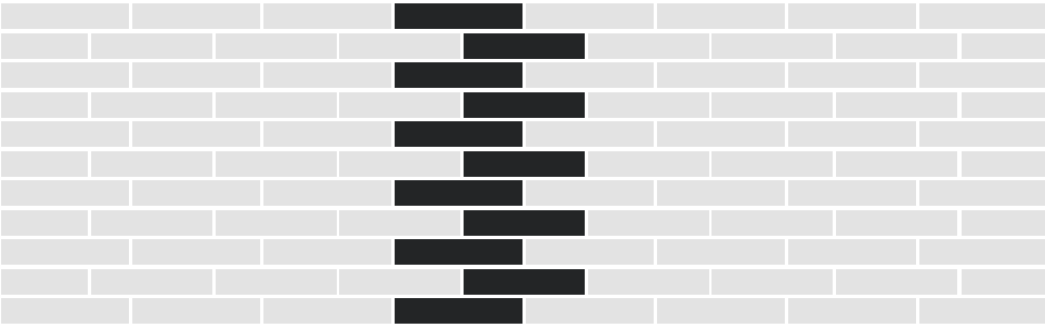
Läuferverband viertel Stein versetzt
