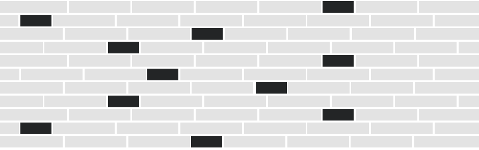
Wild bond
