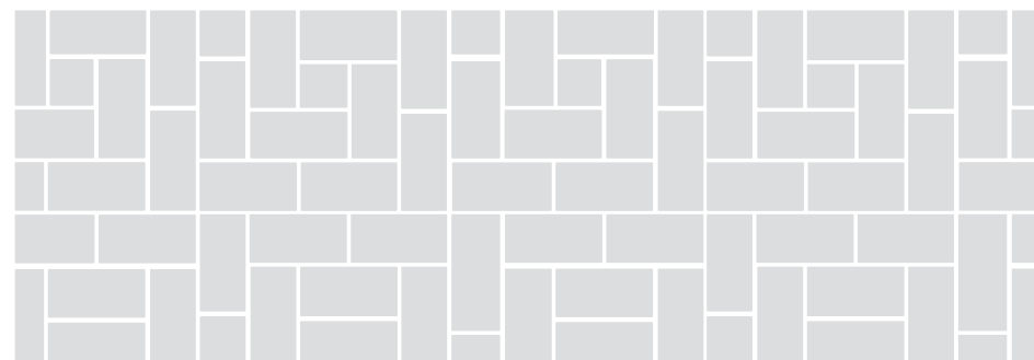
Mittelsteinverband
