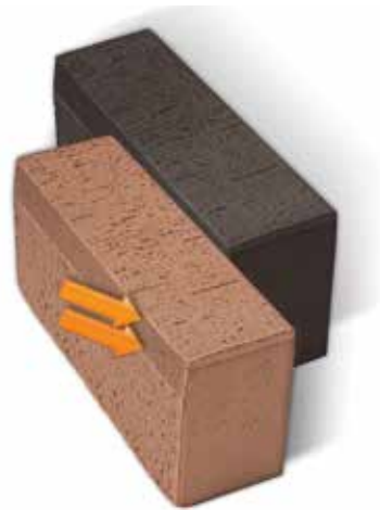
Pflasterklinker mit konischen Abstandhaltern
